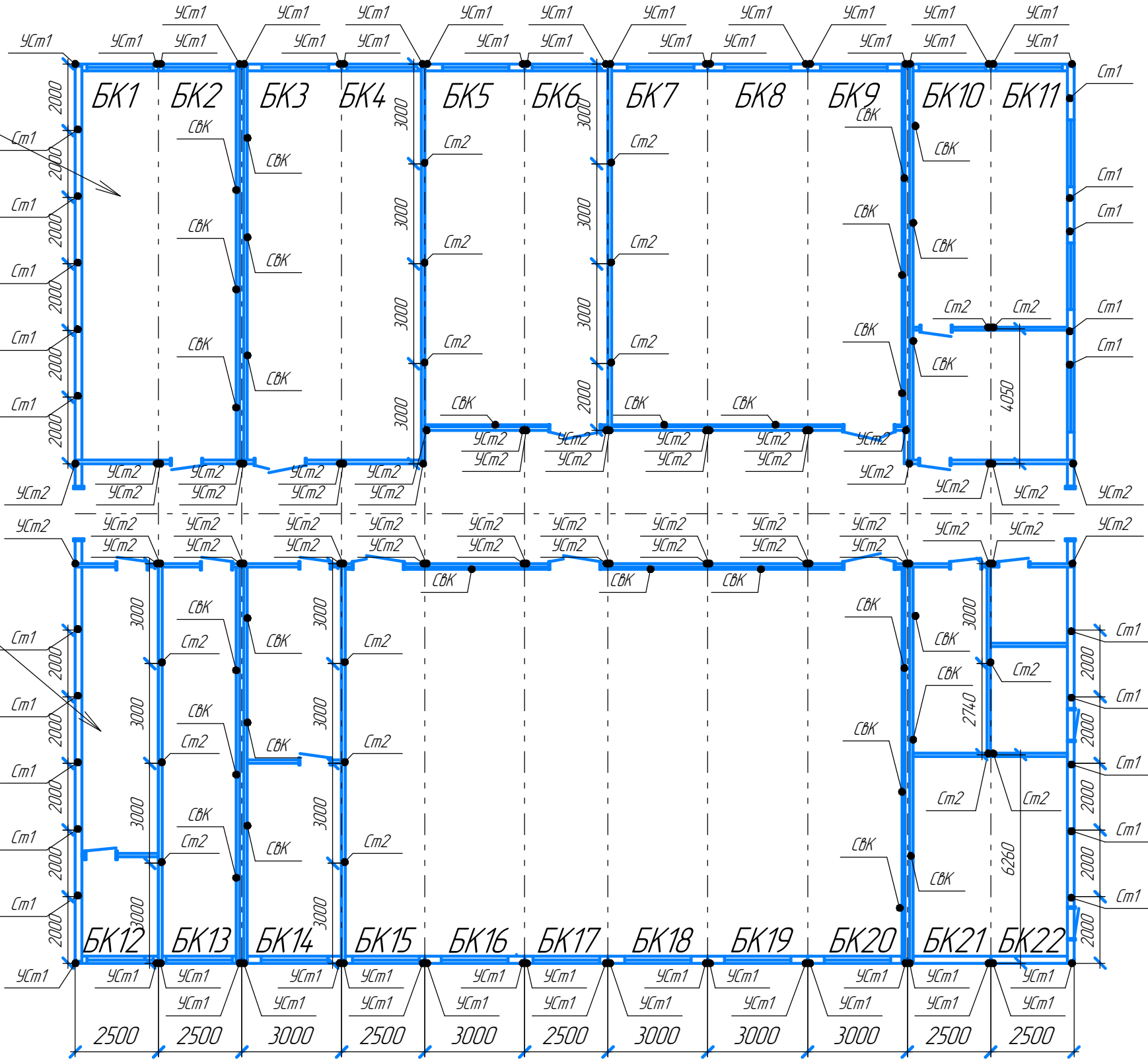
Схема расстановки блок-контейнеров, стоек и связей
